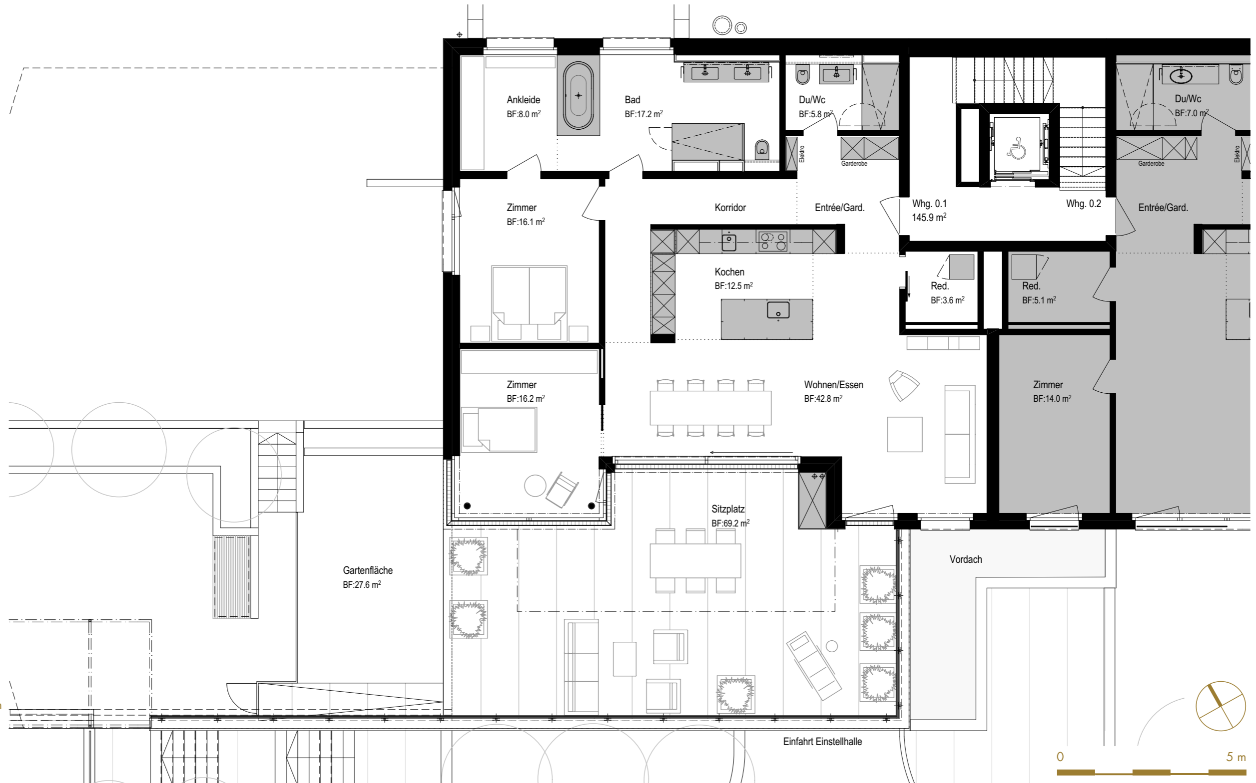
Masstab 1:100
