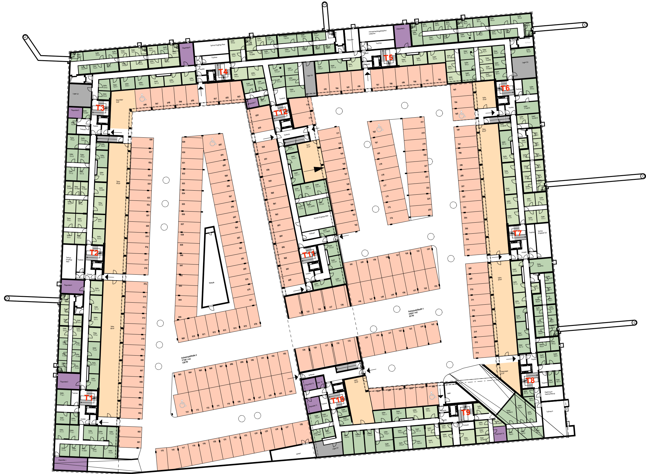
Untergeschoss 1:500
